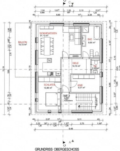
GRUNDRISS OBERGESCHOSS
