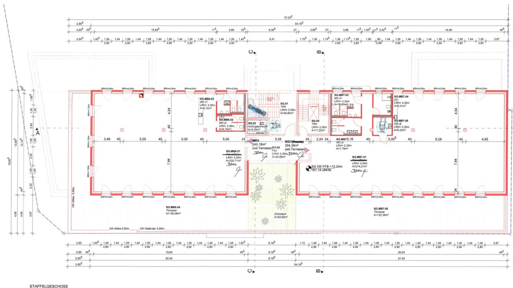
STAFFELGESCHOSS
