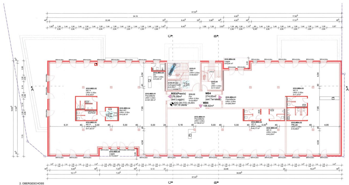
2. OBERGESCHOSS
