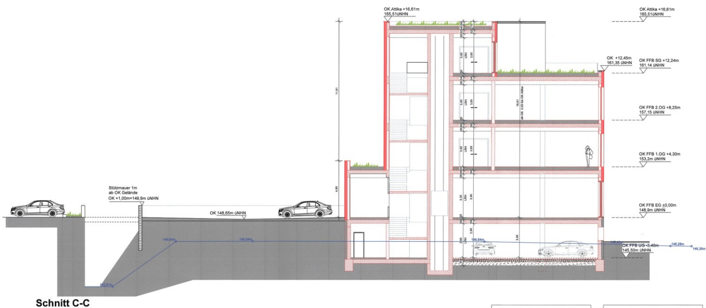
Schnitt C-C
