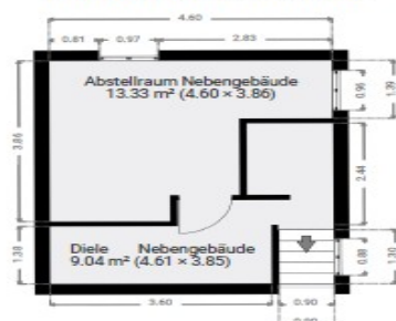
Grundriss Erdgeschoss Nebengebäude
