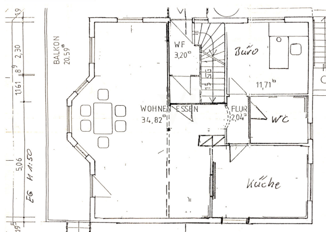
Grundriss EG
