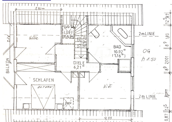
Grundriss OG
