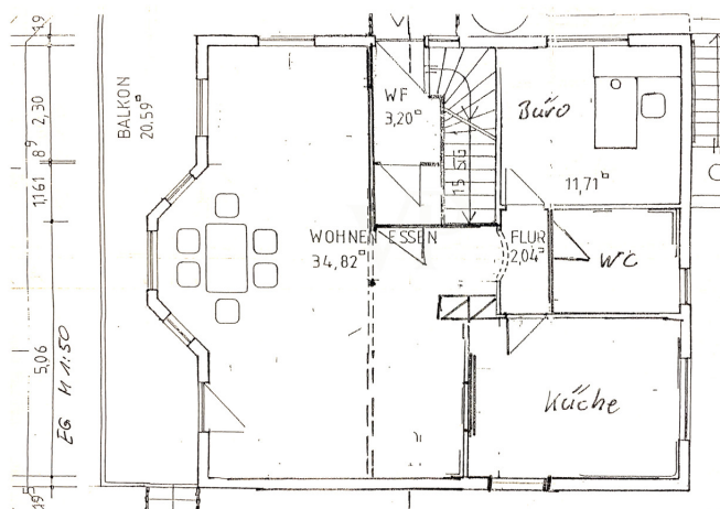
Grundriss EG
