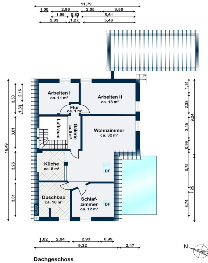
Dachgeschoss
