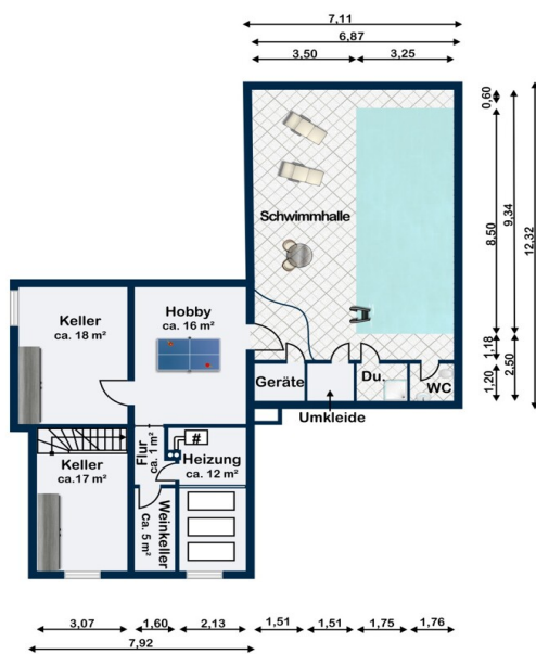
Kellergeschoss
