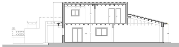
SECCIÓN B-B
