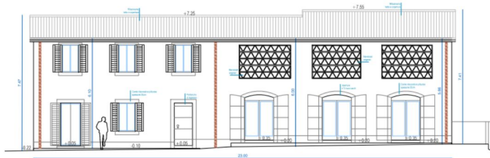
PROSPETTO FRONTE
