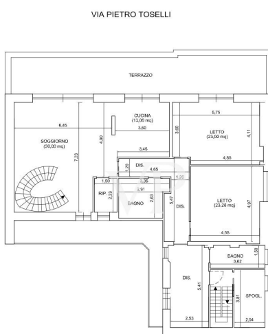
PIANTA PIANO QUARTO H = 3.45 m
