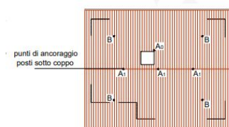
pianta copertura
