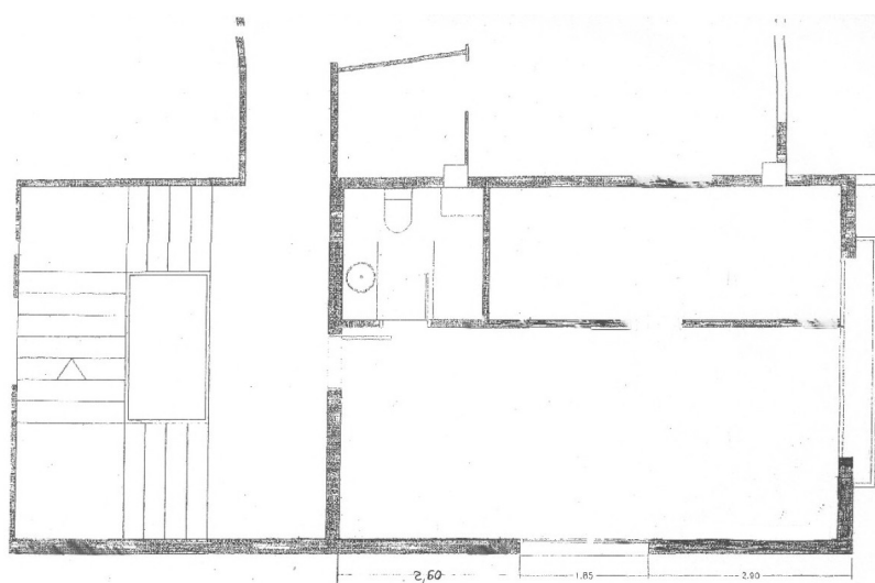
1er Piso
