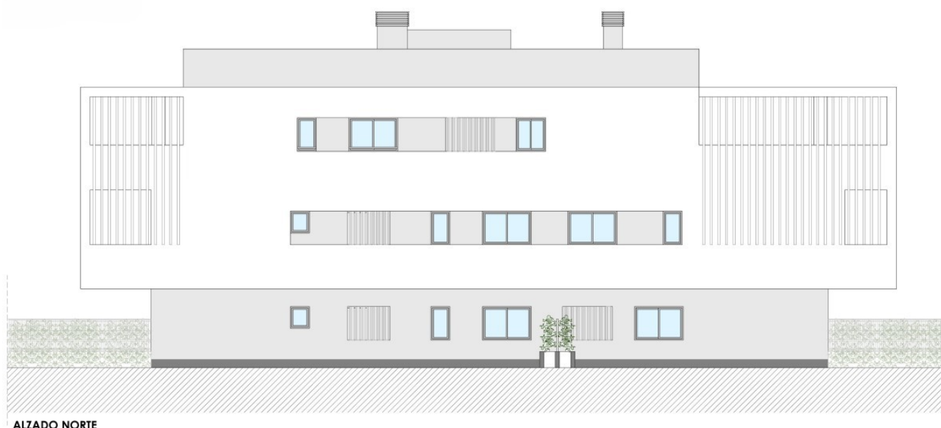
ALZADO NORTE
