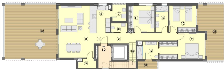
PLANTA SEGUNDA
