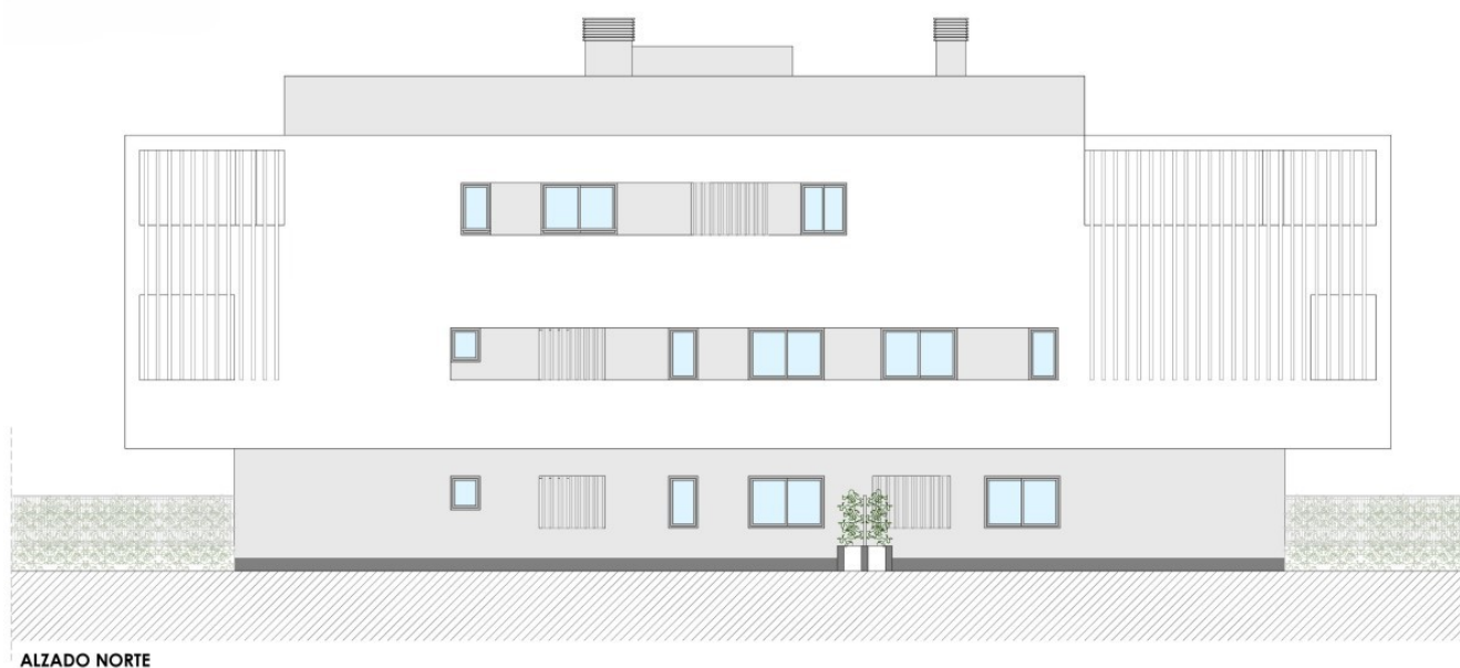
ALZADO NORTE
