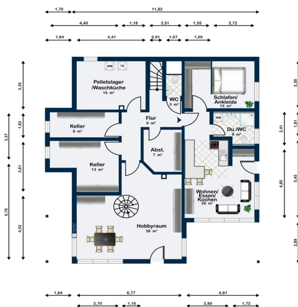
Untergeschoss
