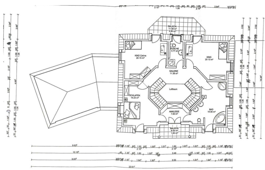
Obergeschoss M 1:100
