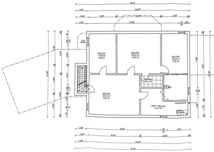
Kellergeschoss M 1:100
