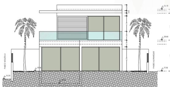
alzado a passeio Violeta 4
