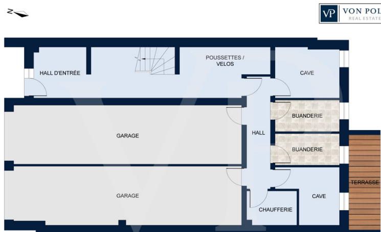
REZ-DE-CHAUSSEE
