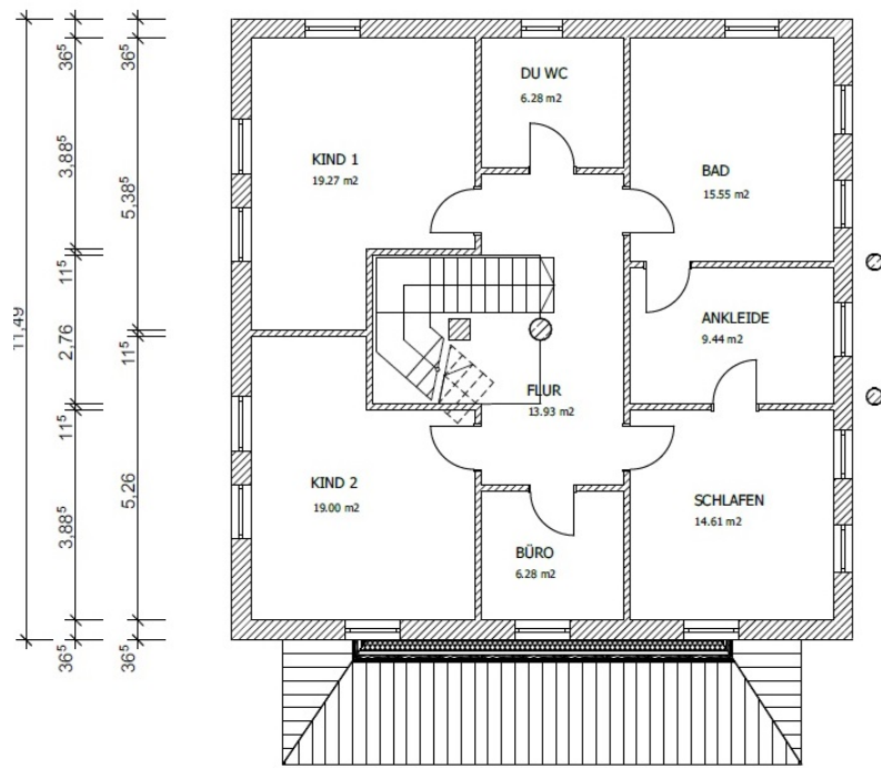
OBERGESCHOSS M 1 : 100
