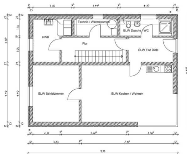
Grundriss Untergeschoss
