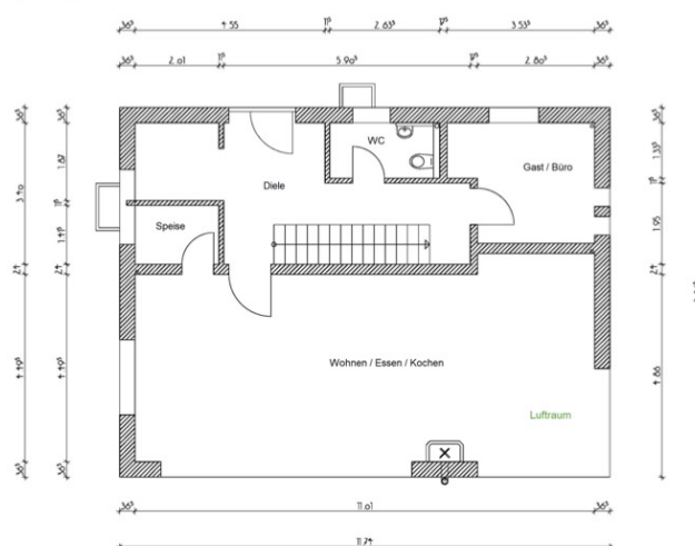
Grundriss Erdgeschoss
