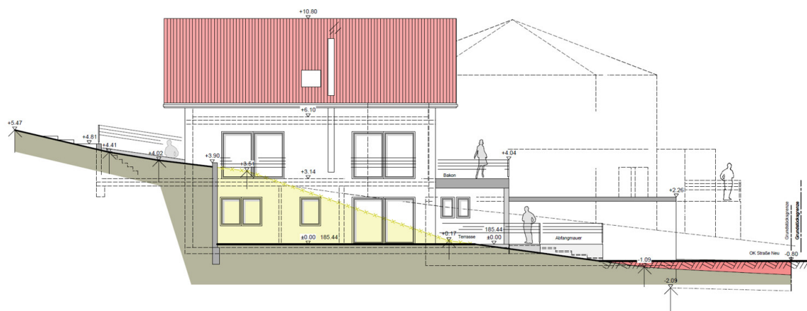
Nordwestansicht 1:100
