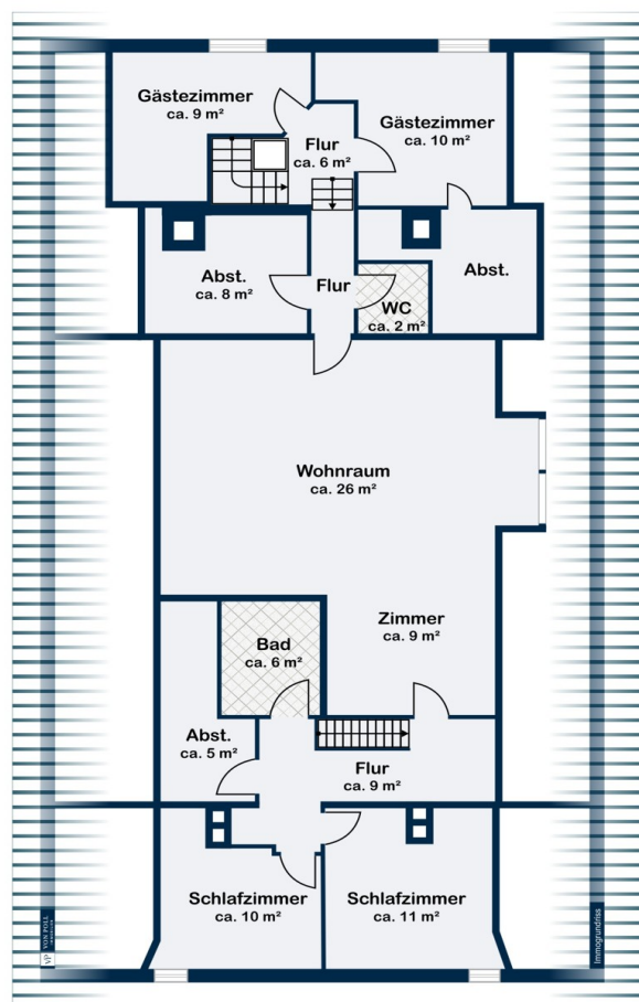
Dachgeschoss
