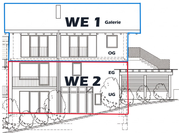
Westansicht
