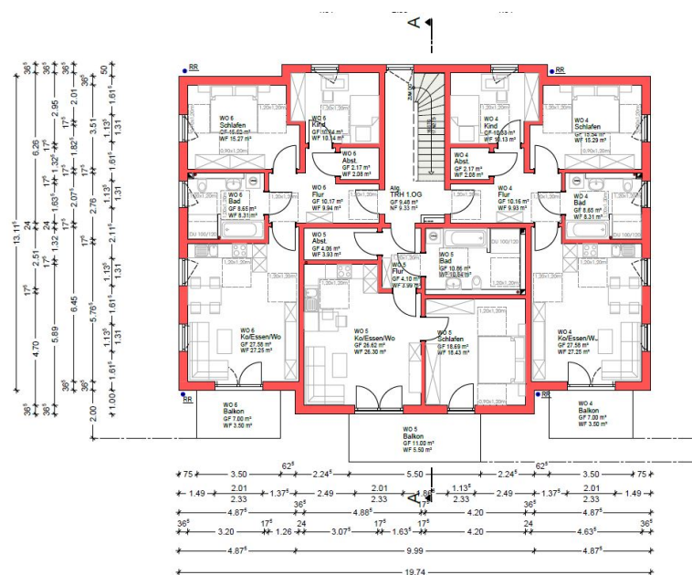
1. Obergeschoss
