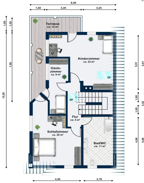
Obergeschoss
