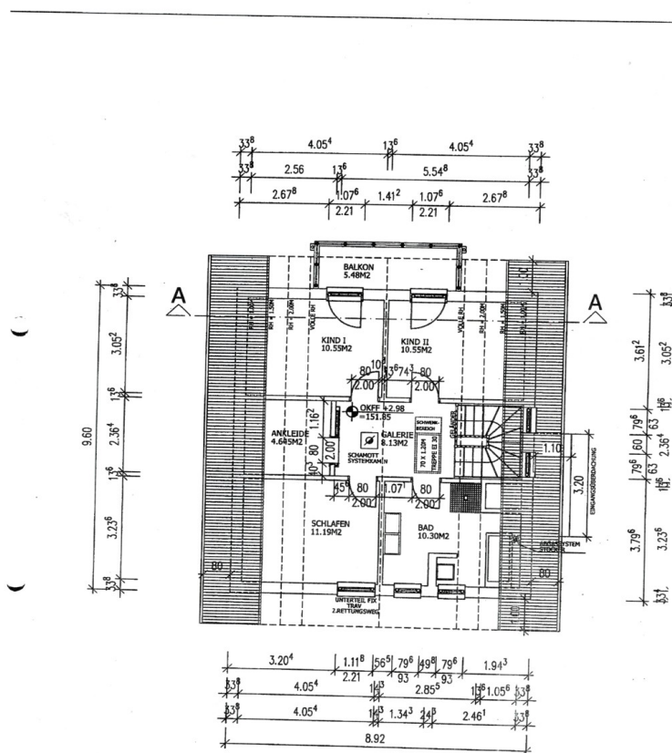
GRUNDRISS OBERGESCHOSS
