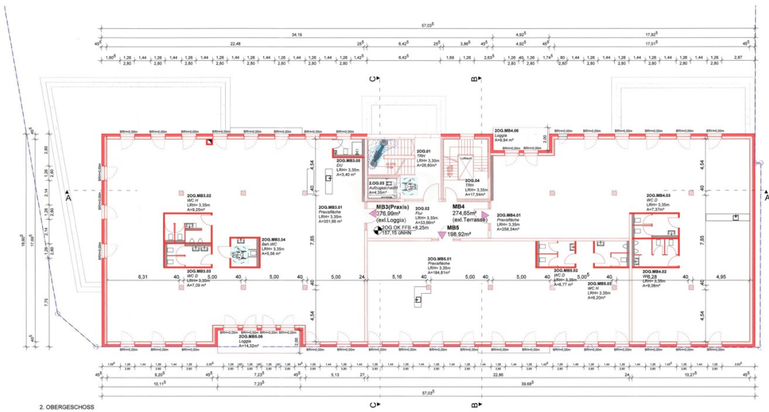
2. OBERGESCHOSS
