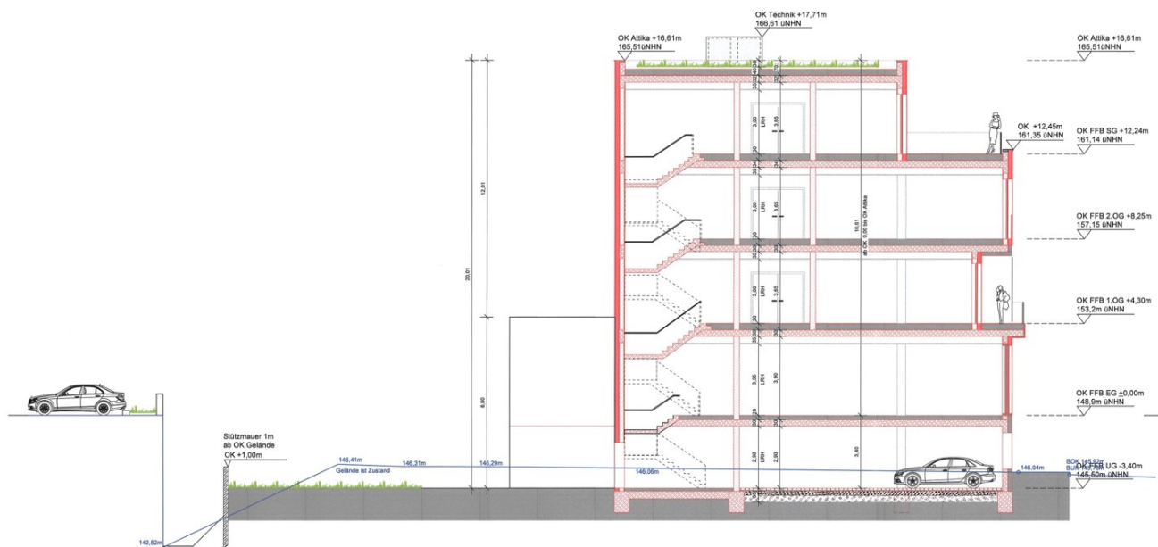
Schnitt B-B
