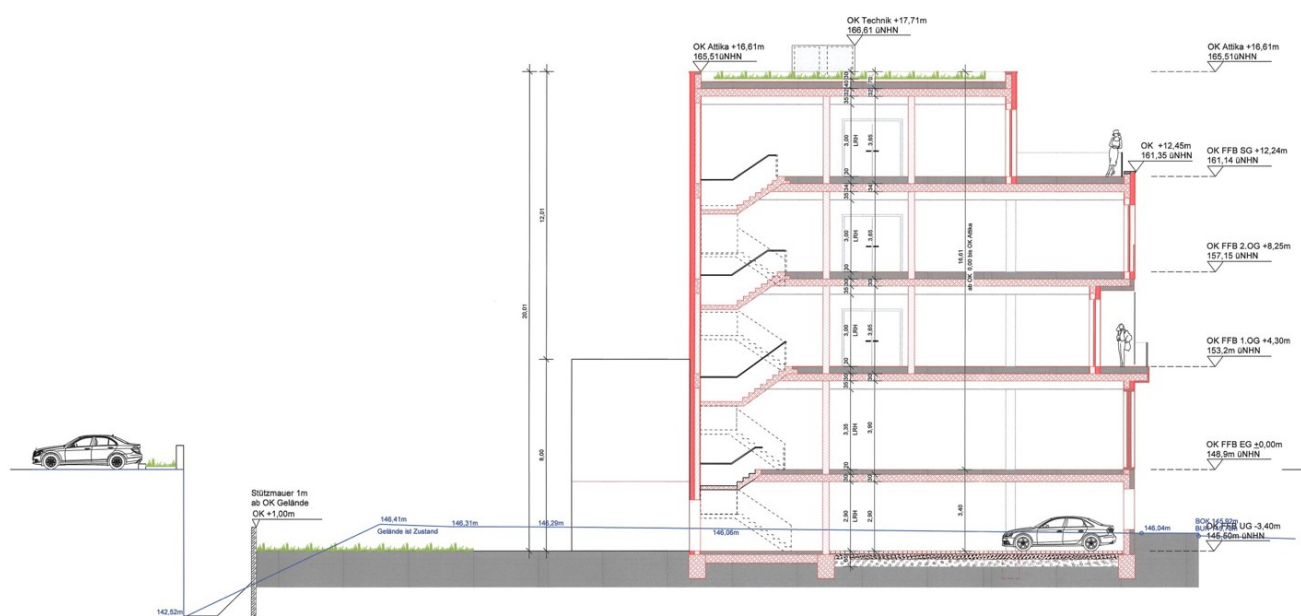
Schnitt B-B
