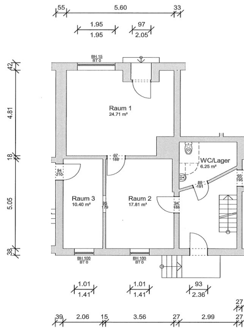
Erdgeschoss: Gewerbe 2
