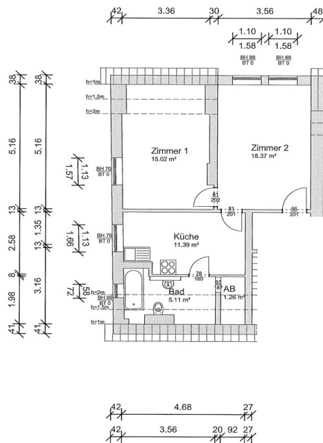
Dachgeschoss: Wohnung 2
