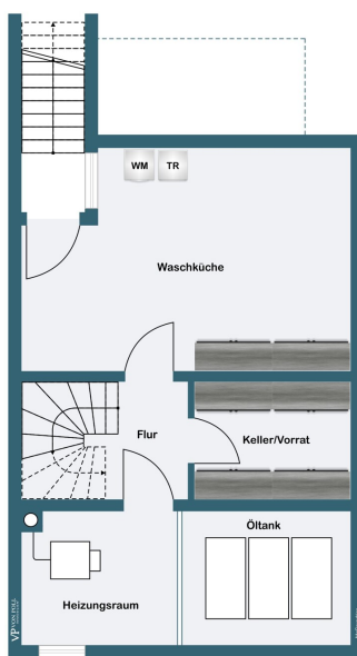
Kellergeschoss
