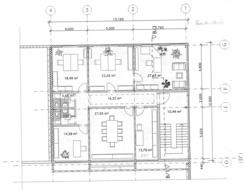
Grundriß Obergeschoß
