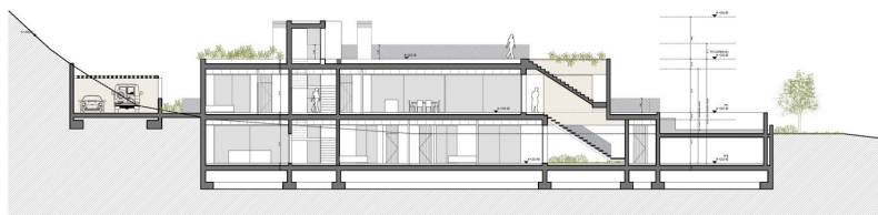
SECCION A-A' # 1/100 000
