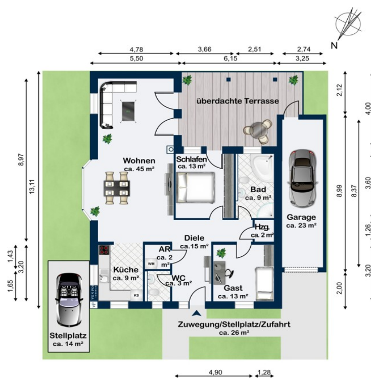
Erdgeschoss
