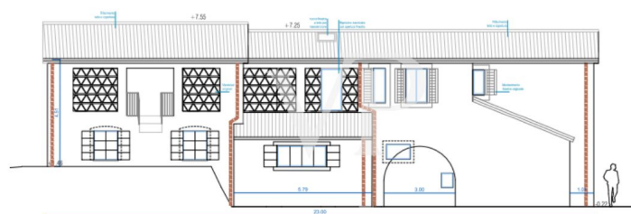
PROSPETTO RETRO
