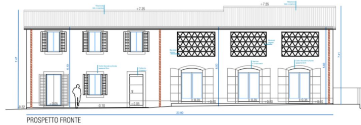
PROSPETTO FRONTE
