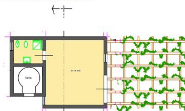
pianta
