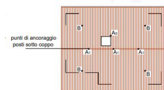
pianta copertura
