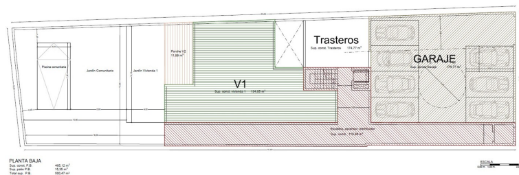
PLANTA BAJA Sup. total P.0 445.12 m² Sup. habit. P.0 16.30 m² Sup. habit. P.0 333.82 m²
