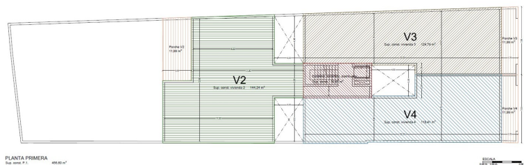
PLANTA PRIMERA Sup. total P.1 445.12 m²
