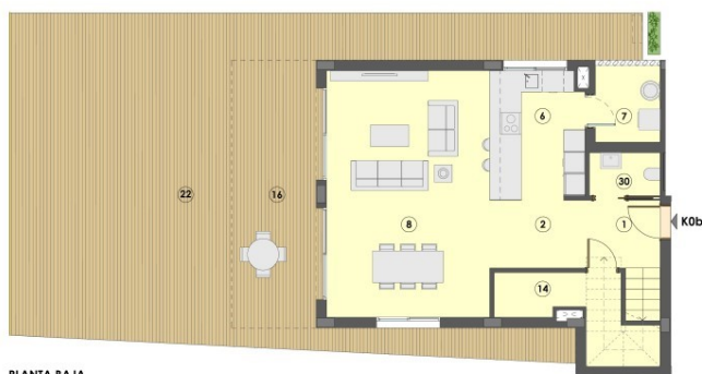
PLANTA BAJA
