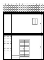
Sezione 3/1 - Sezione trasversale - Edificio proprietà - Edificio proprietà
