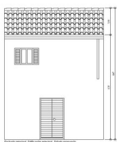
Sezione 1/1 - Sezione trasversale - Edificio proprietà - Edificio proprietà
