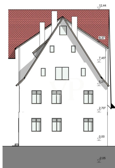
Gebäude J: Ansicht West
