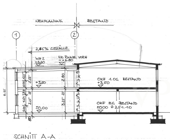
SCHNITT A-A
