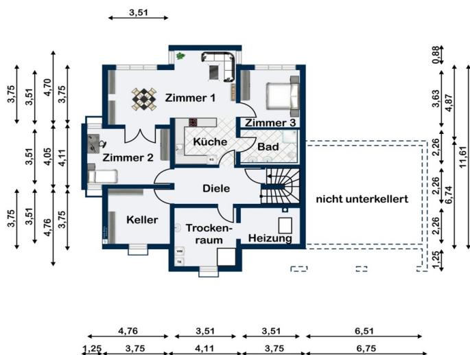
Untergeschoss
