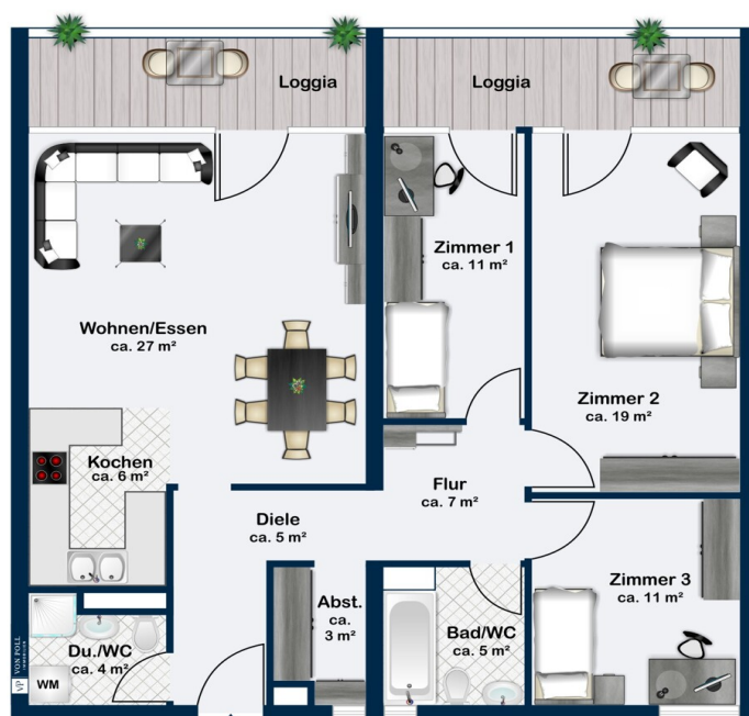
1. Obergeschoss
