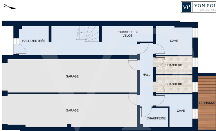
REZ-DE-CHAUSSEE
