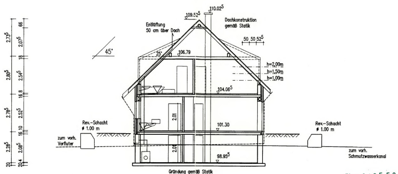
Schnitt A-A
