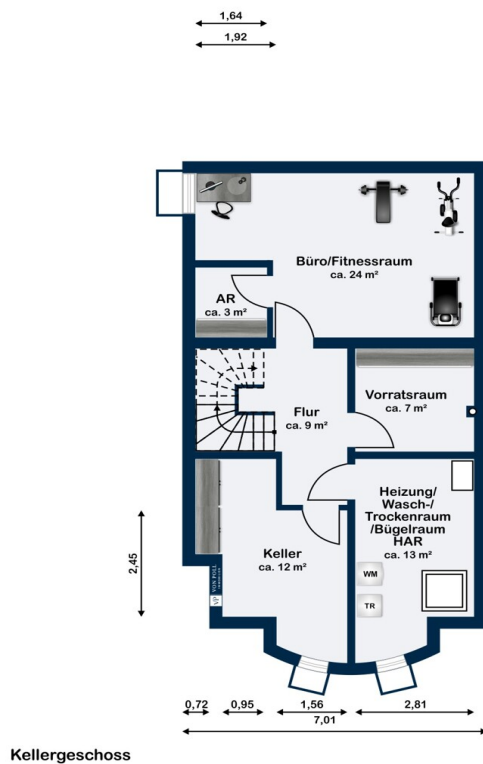
Kellergeschoss
