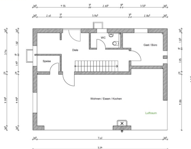
Grundriss Erdgeschoss
